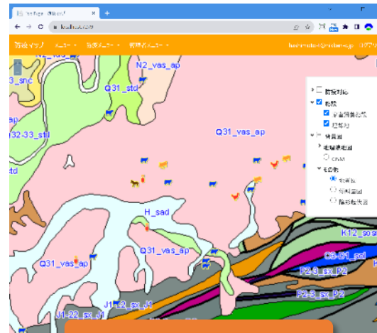
地質図
